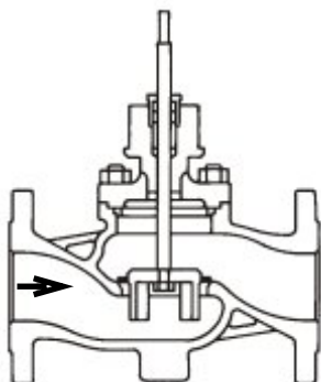
Obr.1: Směr proudění dvoucestnou armaturou s válcovou nebo tvarovanou kuželkou RV 2xx xxx xxxx Lx xx/xxx-xxx (Char. L; R; P; S; U)
