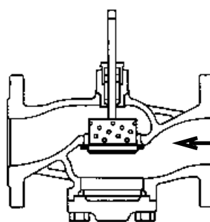
Obr.2: Směr proudění dvoucestnou armaturou s děrovanou kuželkou RV 2xx xxx xxxx Dx xx/xxx-xxx (Char. D; Z; Q)
