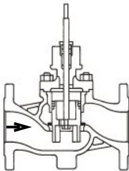
Obr.1: Směr proudění dvoucestnou armaturou s válcovou nebo tvarovanou kuželkou RV 2xx xxx xxxx Lx xx/xxx-xxx (Char. L; R; P; S; U)
