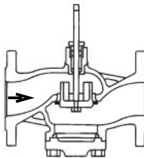
Obr.1: Směr proudění dvoucestnou armaturou s válcovou nebo tvarovanou kuželkou RV 2xx xxx xxxx Lx xx/xxx-xxx (Char. L; R; P; S; U)
