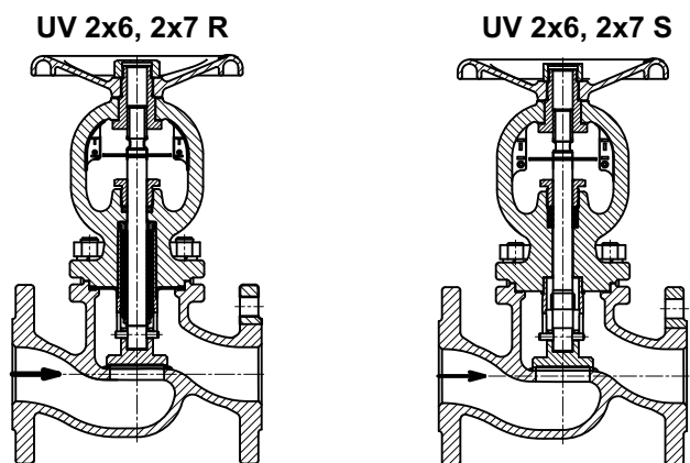
Рис. 1: Направление потока арматуру с тарельчатым или форматированным конусом
