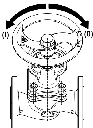
Рис. 3: Маховик-открывать (I), закрывать (0)
