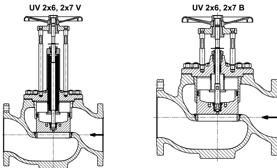
Рис. 2: Направление потока арматуру с разгруженным по давлению конусом
